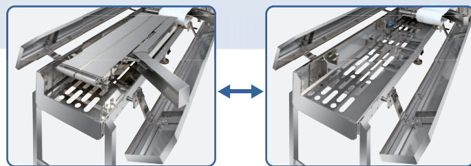
供給コンベアベルト脱着式 (工具不要)
